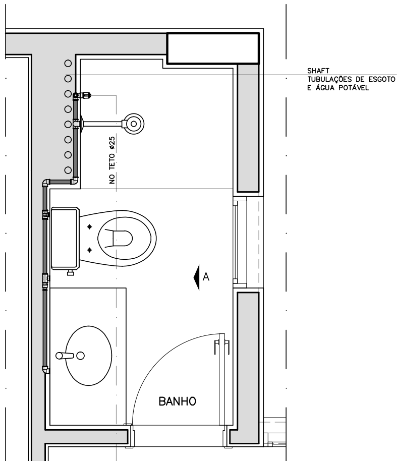
PLANTA BAIXA ESC._1/25
